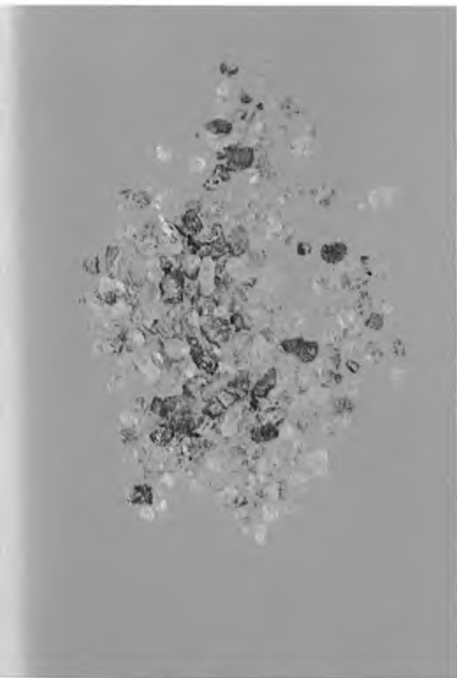
Olivina
